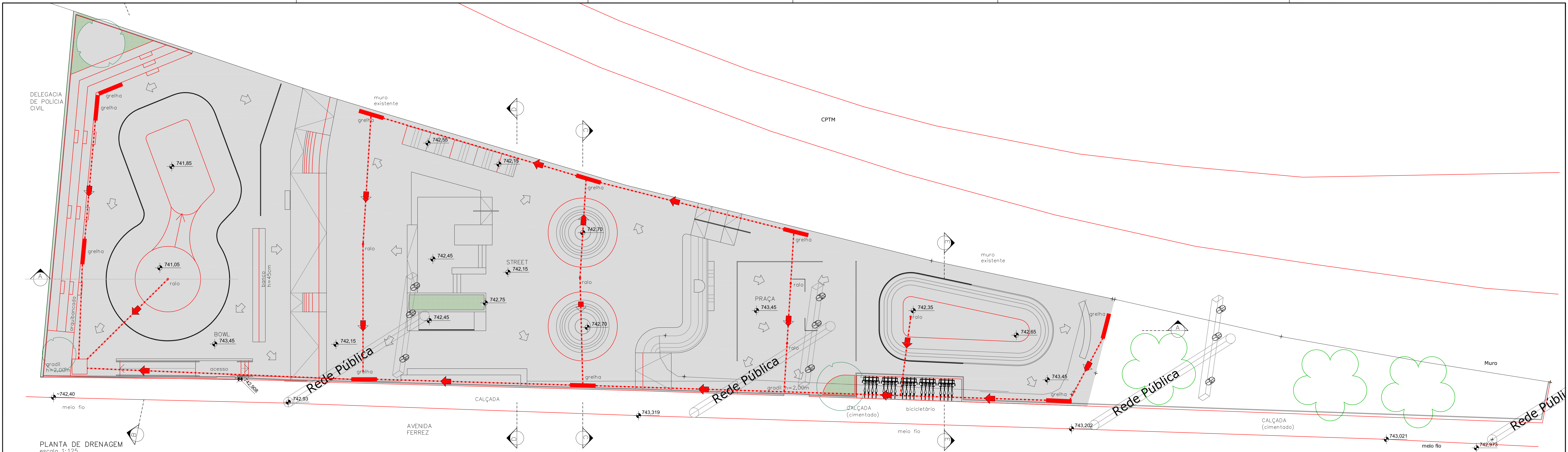
PLANTA DE DRENAGEM escala 1:125 → caminhamento tubulação de águas pluviais
