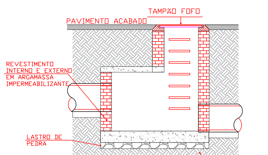
CORTE AA – POÇO DE VISITA
