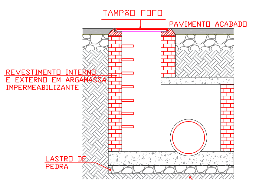
CORTE BB – POÇO DE VISITA
